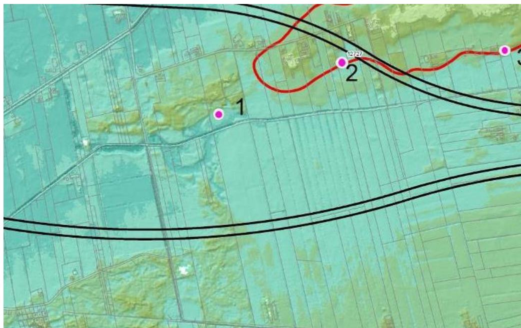
Laagte bij Varsenerveld die duid op een oude rivierarm (vergroting van figuur pag. 4)
